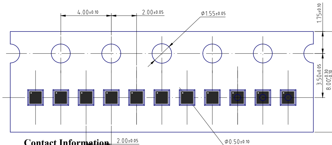
DFN1x1-4L
