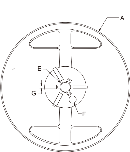
Reel (7")
