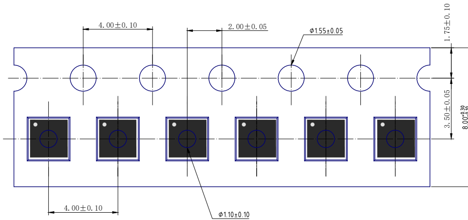
DFN1x1-4L
